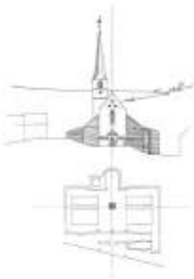
Neuer, geplanter Erweiterungsentwurf der Pfarrkirche St. Barbara, Wismarstadt und Grundriss. Architekt: Dipl.-Ing. Hans-Joachim Wacker, Wismar
